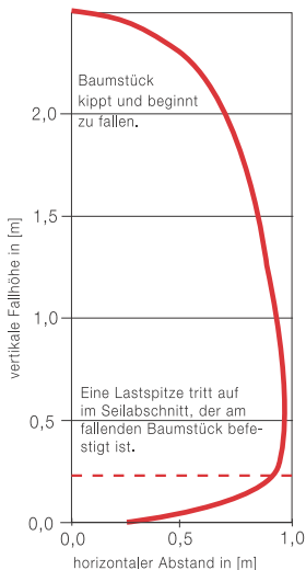
Fallkurve des Schwerpunktes
